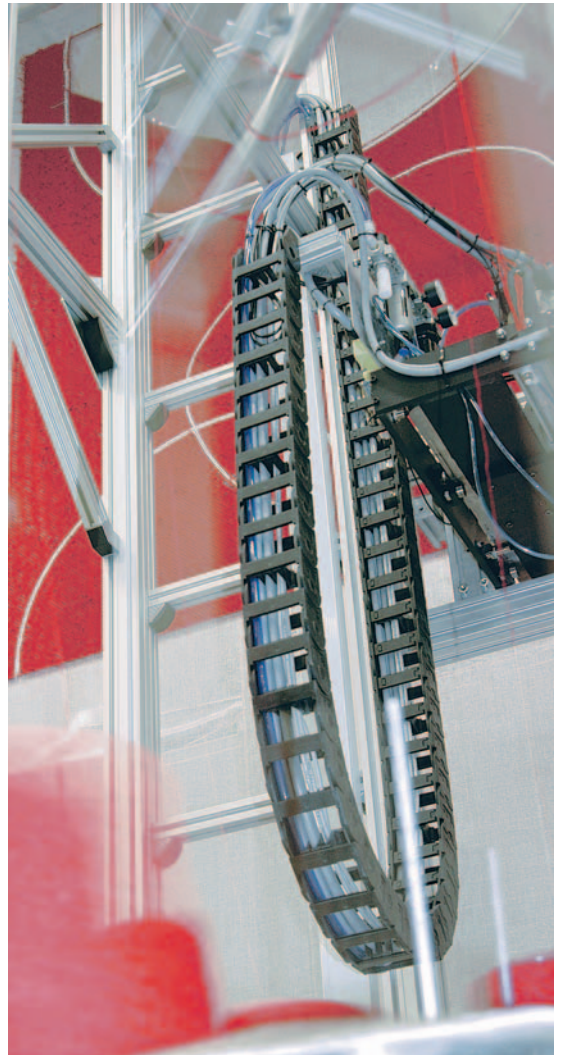
Teppichknüpf-Roboter Rug-making robot Robot pour nouage de tapis Hitex AB, Svängsta, S
